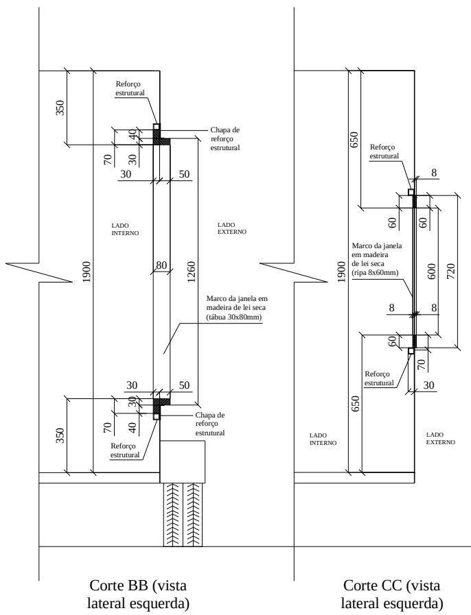
Figura C.6 - Detalhe para instalação das molduras de madeira: Corte BB e CC - vista lateral esquerda (sem escala)
