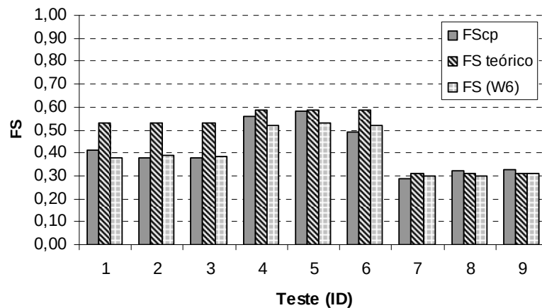
Quadro 7-3. Resumo das comparações entre FS (proteções internas)
