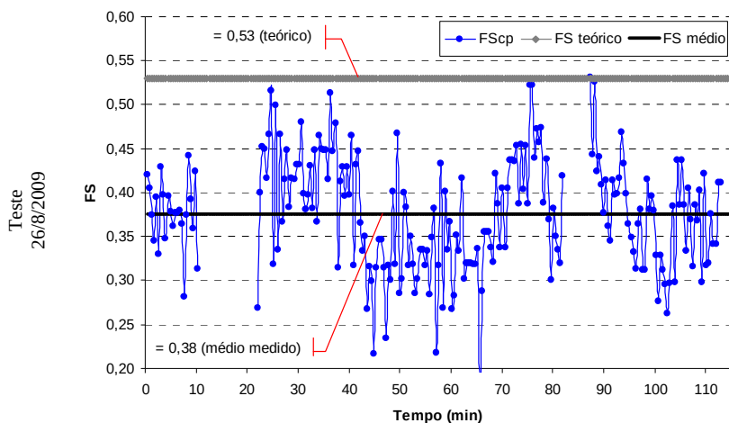
Quadro 6-9. Resultados de FS medido na CP (persiana horizontal - preta - 45°)
