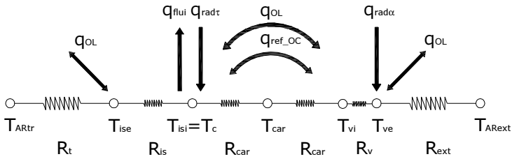
Figura G.1. Equivalente eléctrico para a CP
