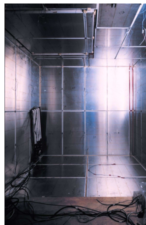
Figura 2-11. Interior de uma das câmaras (LBNL, 2007)
