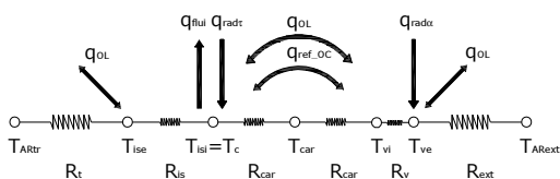
Equivalente elétrico
