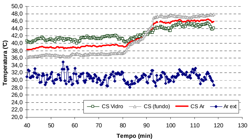
Figura 4-14. Variação de temperatur na CS (segundo teste)
