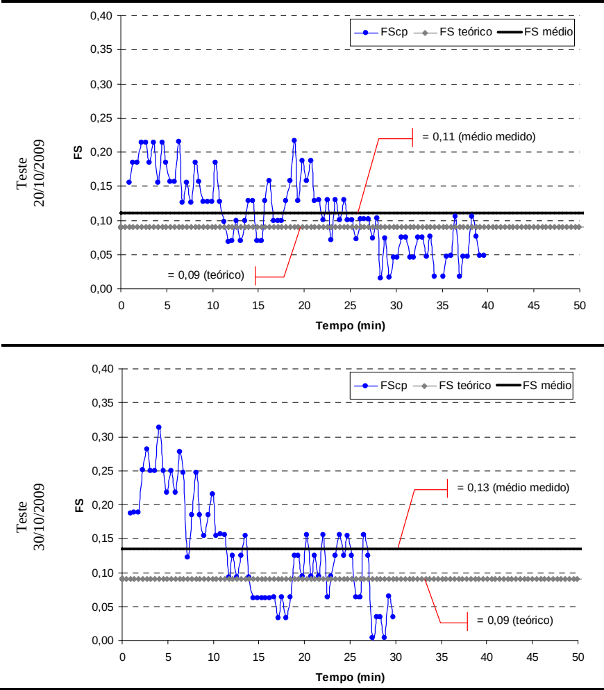
Quadro 6-12. Resultados de FS medido na CP (brise horizontal branco - 45°) – banho “off”
