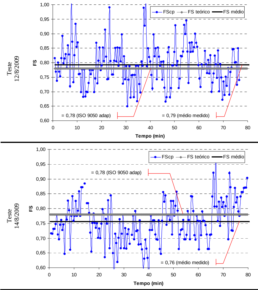
Quadro 6-5. Resultados de FS medido na CP (vidro incolor 6mm)
