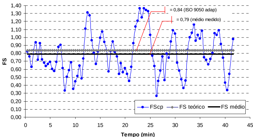
Figura 4-7. Fator solar medido no primeiro teste de calibração (ângulo de incidência \sim 45^\circ ) 8
