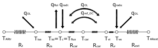
Equivalente elétrico
