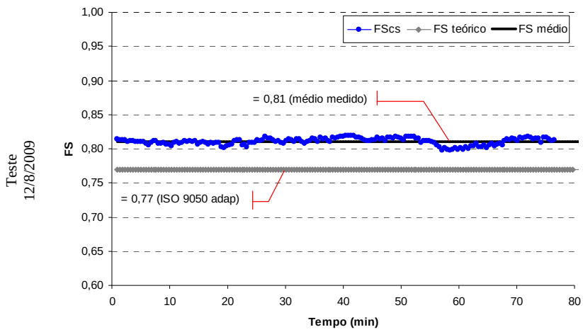
Quadro 6-6. Resultados de FS medido na CS (vidro incolor 6mm)
