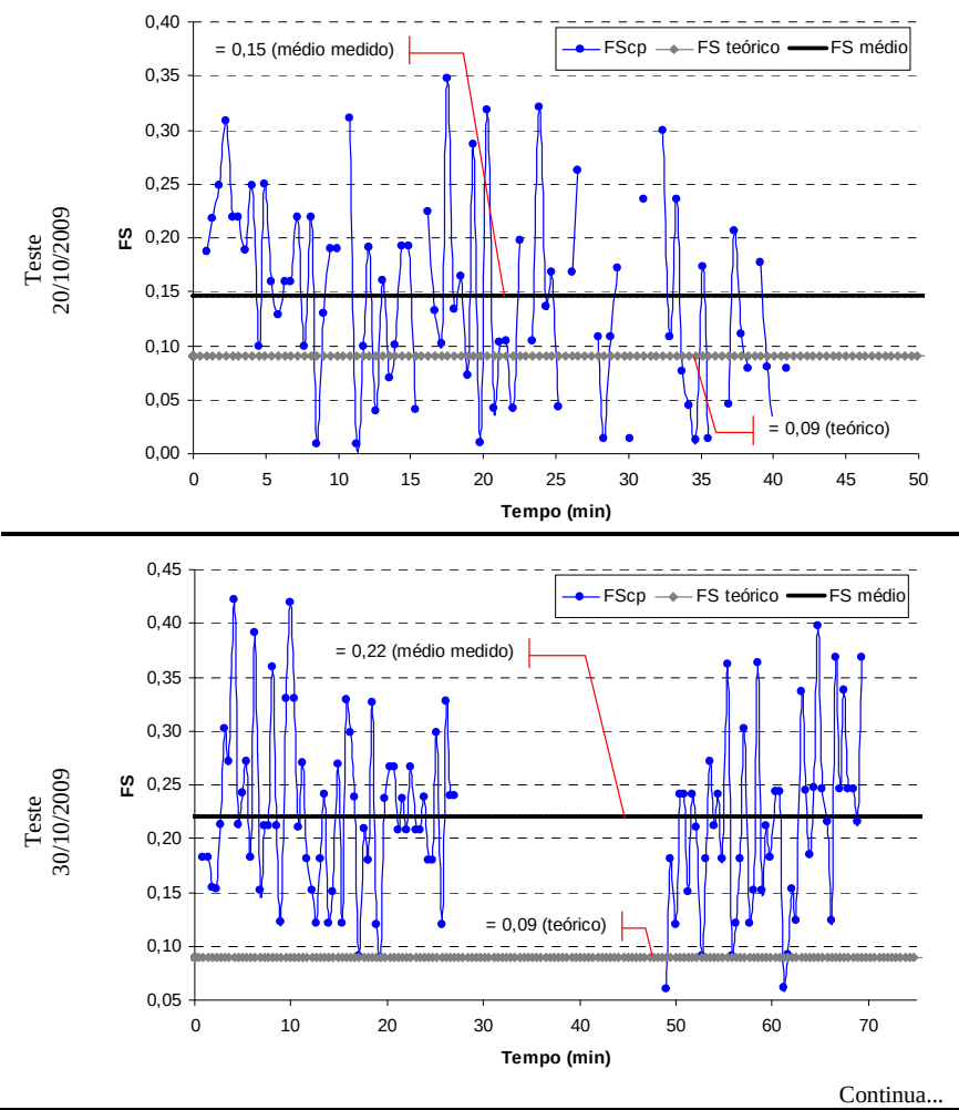
Quadro 6-13. Resultados de FS medido na CP (brise horizontal branco - 45°) – banho “on”
