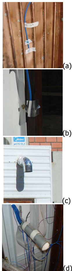
Figura 3-50. Exemplo da fixação dos termopares (a); exemplo de proteção dos termopares quando expostos à radiação solar (b); entrada para medição da temperatura do ar (c); junta de referência dos termopares (d)
