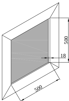
Figura 3-2. Desenho esquemático da cavidade de secundária (cotas em mm)
