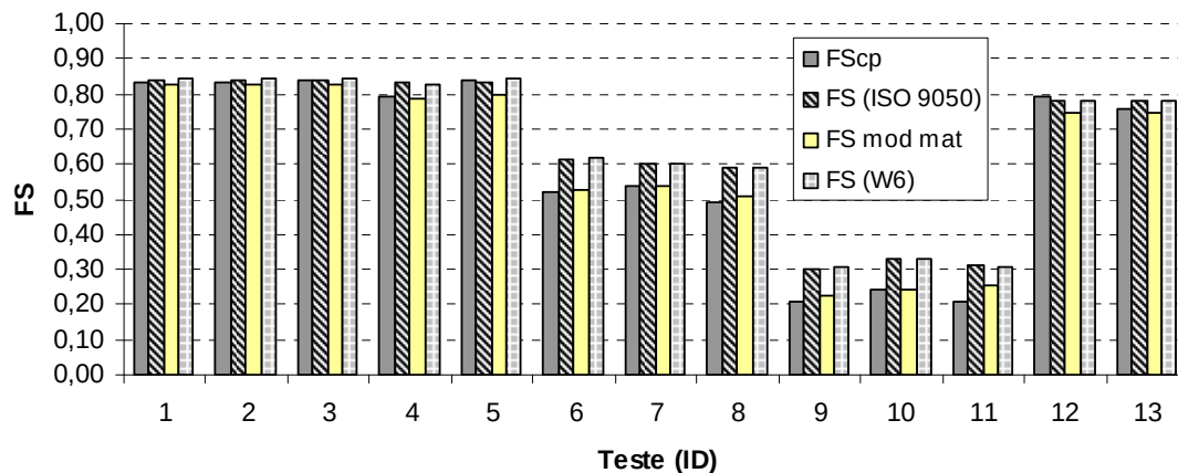
Quadro 7-1. Resumo das comparações entre FS (vidros na CP)
