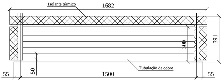
Vista Superior
