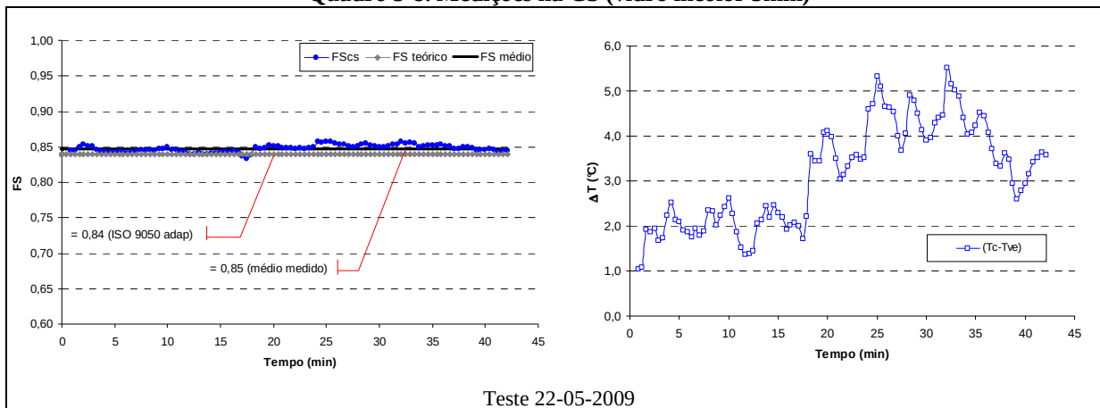
Quadro 5-8. Medições na CS (vidro incolor 3mm)
