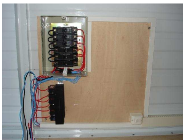
Figura 3-28. Quadro de distribuição elétrica
