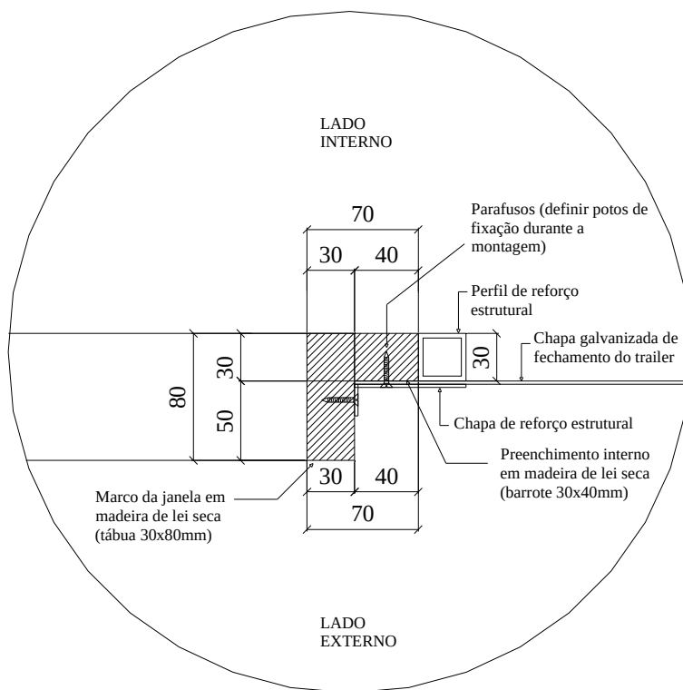
Figura C.7 - Detalhe de fixação da moldura de madeira: marco da abertura da cavidade principal (sem escala)
